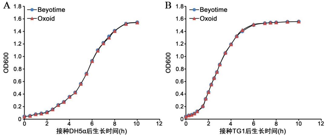
图1. 碧云天的BeyoPure™胰蛋白胨和BeyoPure™酵母膏配制的LB培养液与用国外Oxoid的胰蛋白胨和酵母膏配制的LB的细菌培养效果图。上图为大肠杆菌DH5α(A)和TG1(B)在碧云天和Oxoid产品配制的LB培养液中的生长曲线比较。
